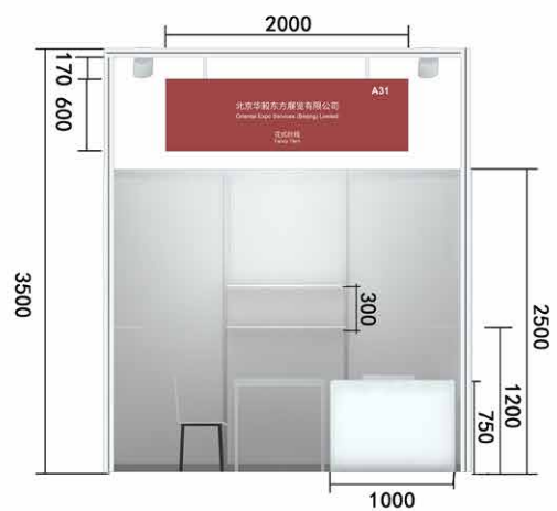
立面图
